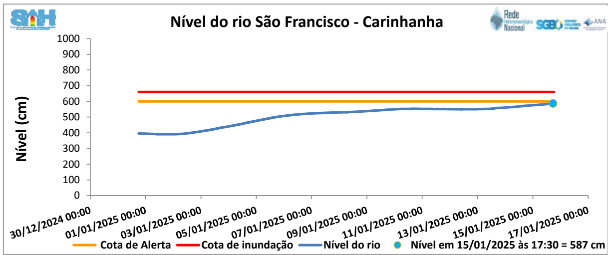
Figura 8. Nível do rio São Francisco na estação de Carinhanha no município de Carinhanha nos últimos 15 dias
