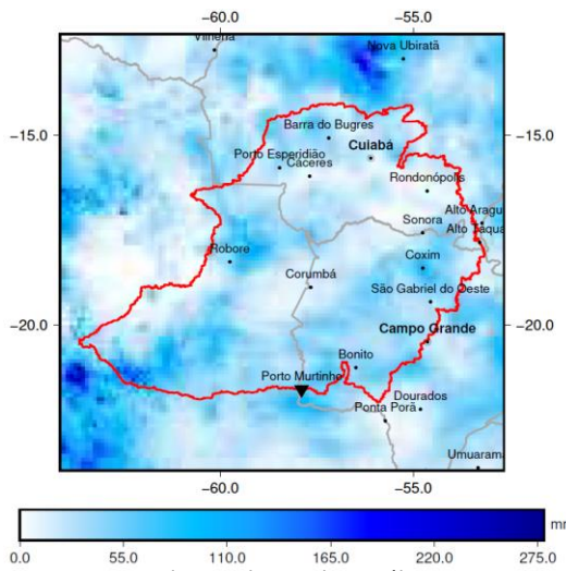
Figura 16. Chuvas observadas na última semana na bacia do Rio Paraguai delimitada à jusante pela estação de Porto Murtinho (34 mm).
