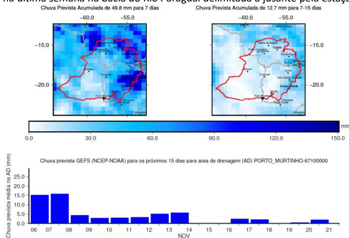
Figura 17. Média da previsão de 21 membros do Ensemble do GEFS/NOAA (63 mm para as próximas duas semanas).
