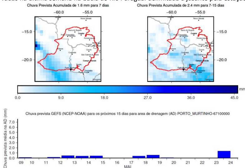
Figura 17. Média da previsão de 21 membros do Ensemble do GEFS/NOAA (4 mm para as próximas duas semanas).
