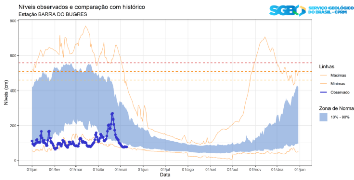
Figura 2. Últimos dados e comparação com o histórico sazonal na estação BARRA DO BUGRES no RIO PARAGUAI.
