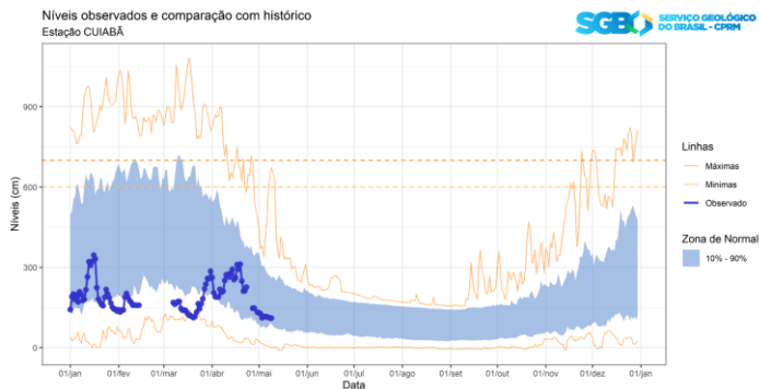
Figura 4. Últimos dados e comparação com o histórico sazonal na estação CUIABÁ no RIO CUIABÁ.
