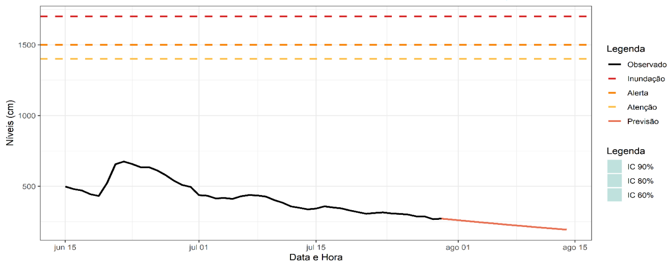
Figura 4. Previsão de níveis em Porto Velho com o modelo SMAP utilizando a previsão de precipitação por ensemble a partir do modelo GEFS.
