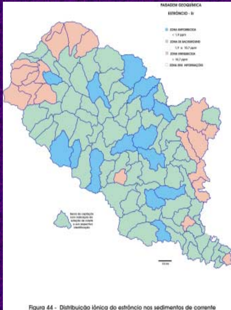
Figura 44 - Distribuição iônica do estrôncio nos sedimentos de corrente
