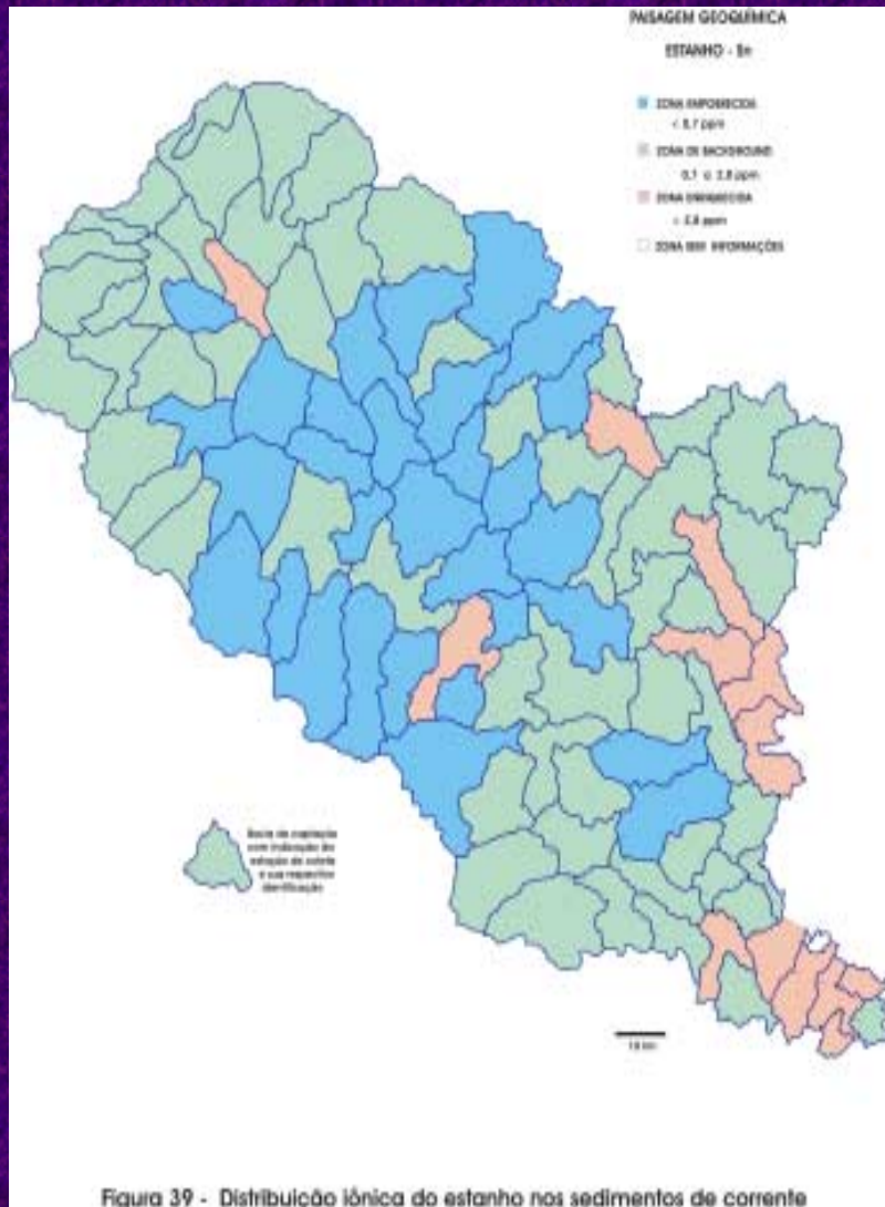
Figura 39 - Distribuição iônica do estanho nos sedimentos de corrente
