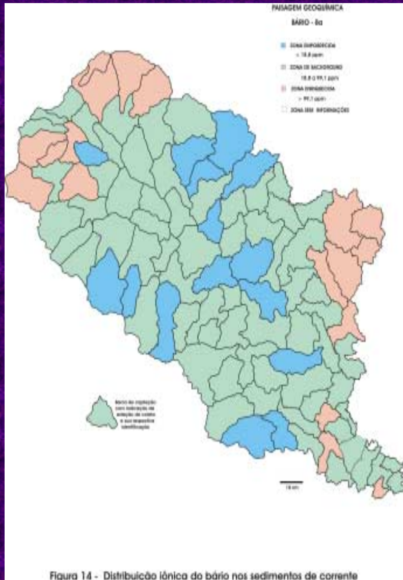
Figura 14 - Distribuição iônica do bário nos sedimentos de corrente
