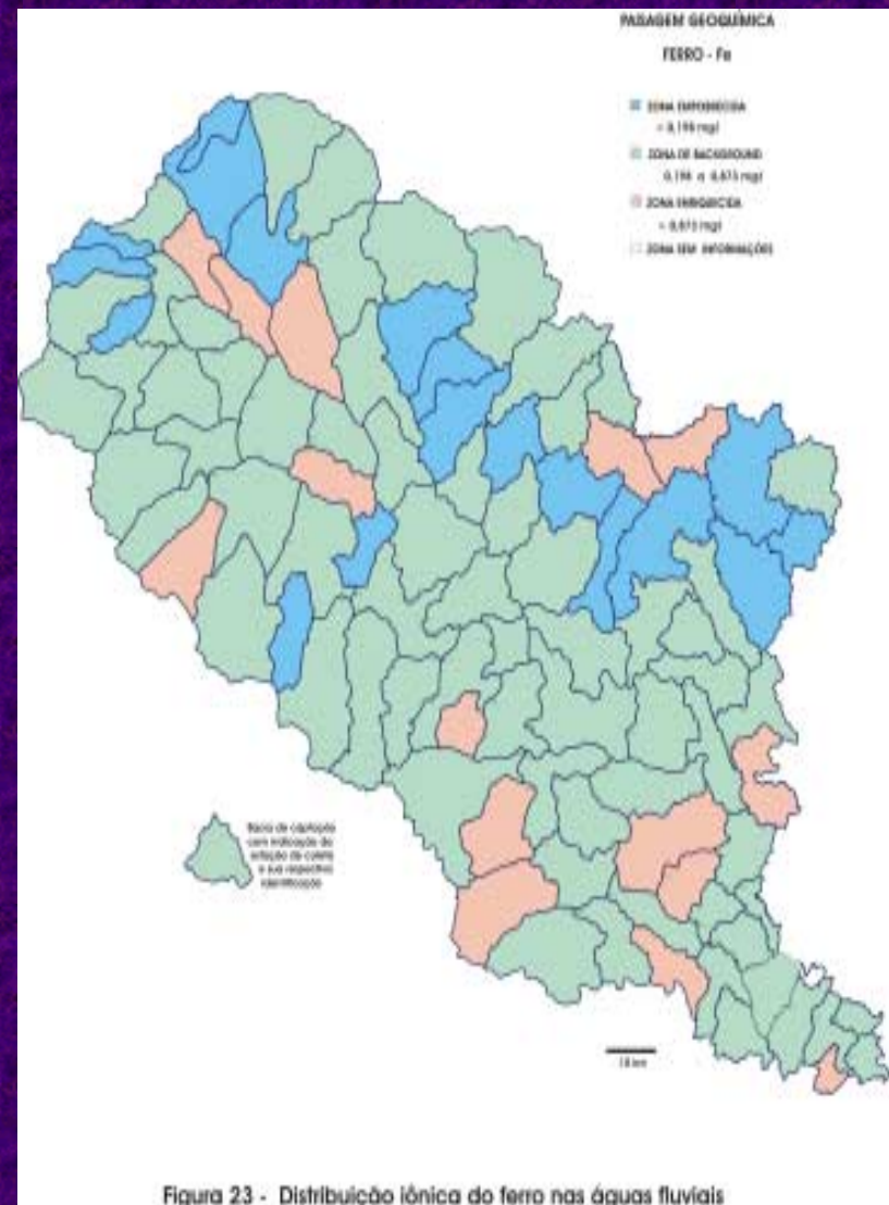
Figura 23 - Distribuição iônica do ferro nas águas fluviais
