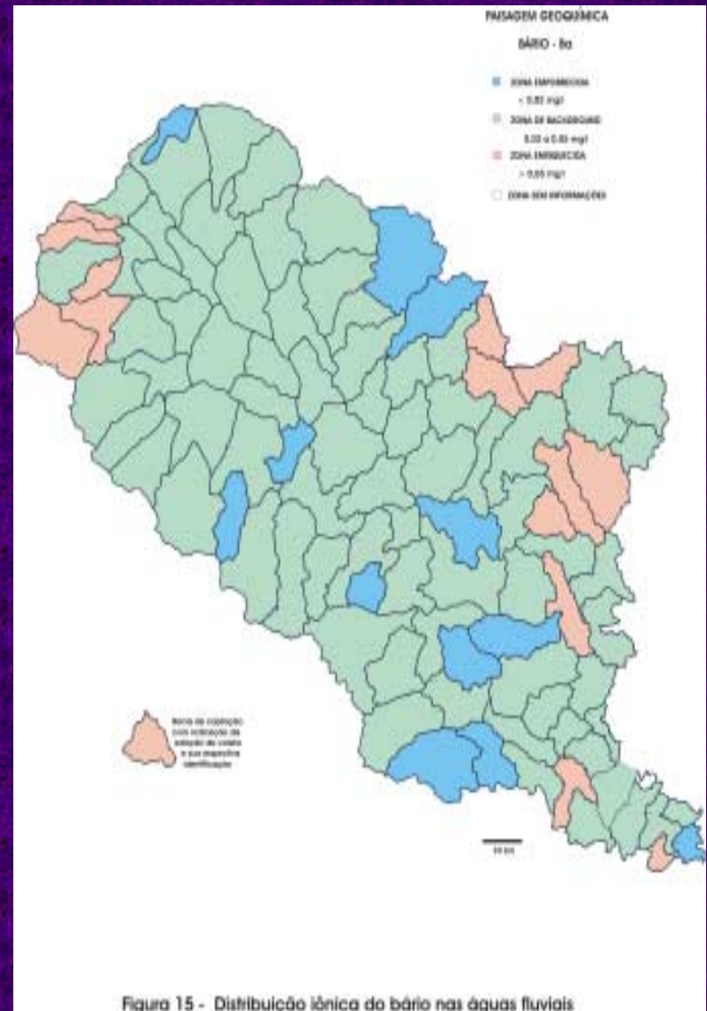
Figura 15 - Distribuição iônica do bário nas águas fluviais
