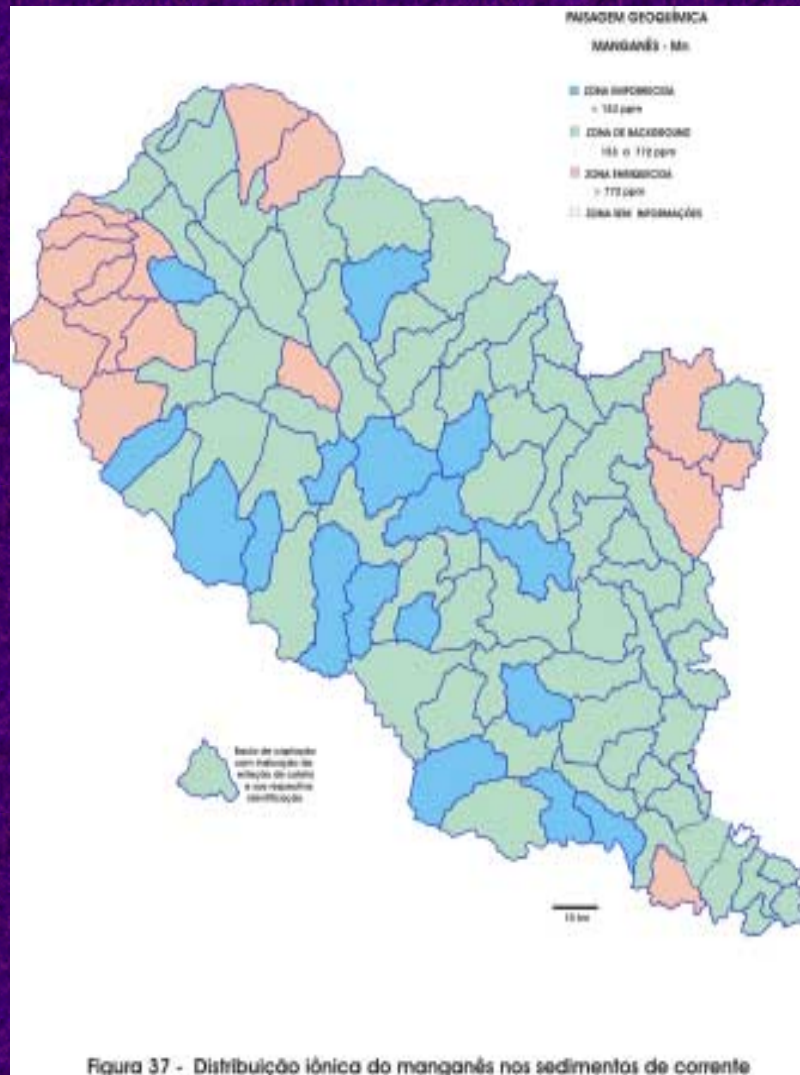
Figura 37 - Distribuição iônica do manganês nos sedimentos de corrente
