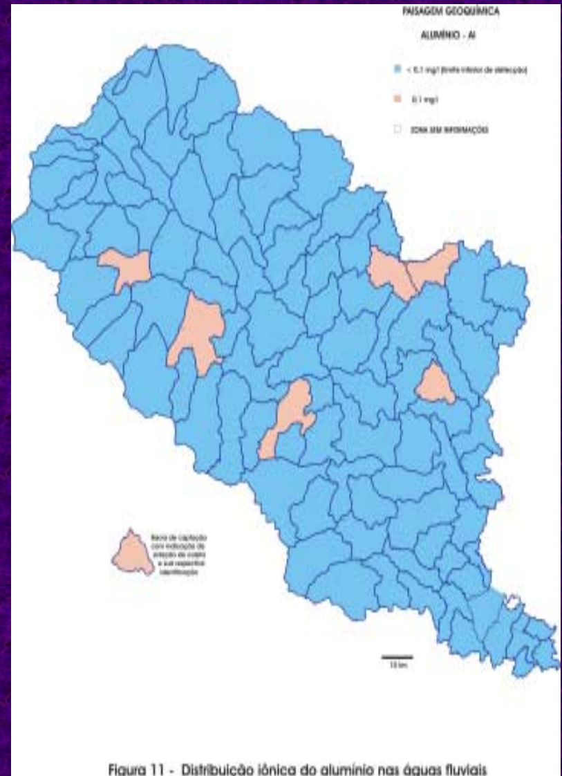
Figura 11 - Distribuição iônica do alumínio nas águas fluviais
