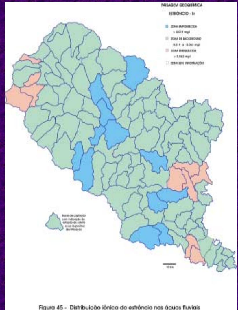
Figura 45 - Distribuição iônica do estrôncio nas águas fluviais
