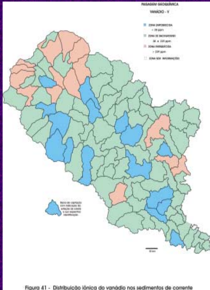
Figura 41 - Distribuição iônica do vanádio nos sedimentos de corrente
