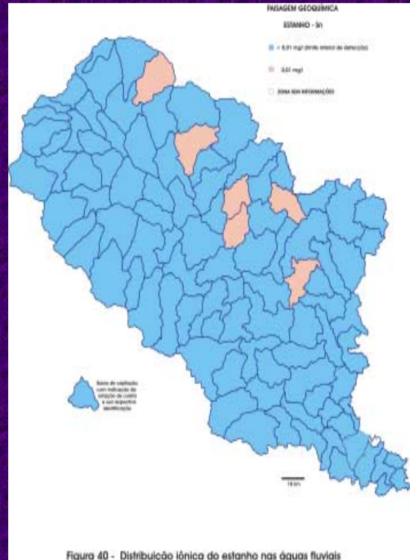
Figura 40 - Distribuição iônica do estanho nas águas fluviais
