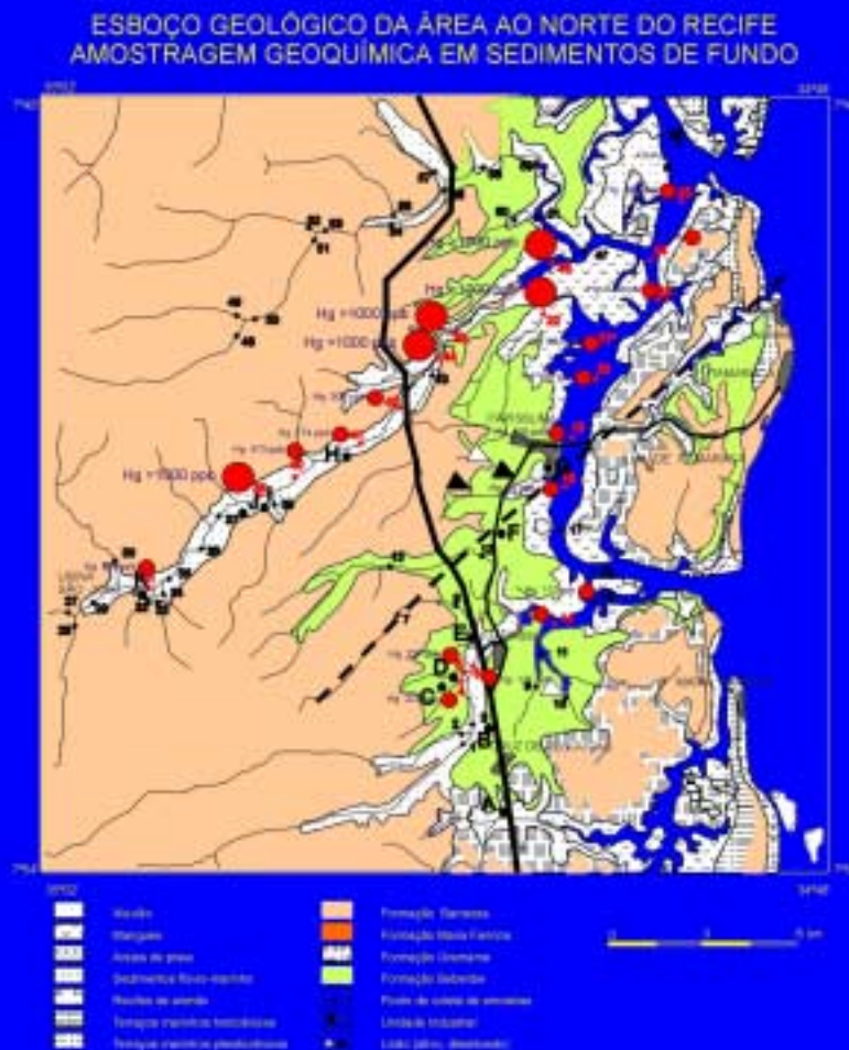
DISTRIBUIÇÃO DE MERCÚRIO EM DRENAGENS
