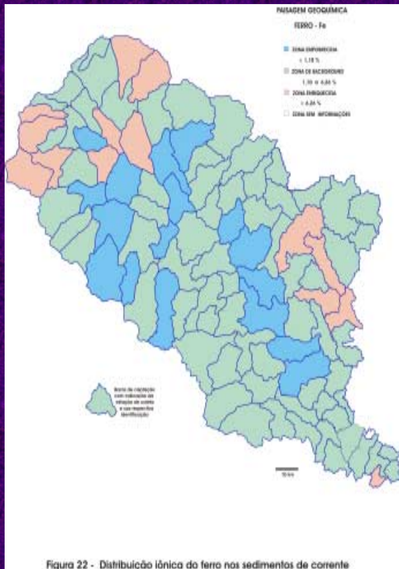
Figura 22 - Distribuição iônica do ferro nos sedimentos de corrente
