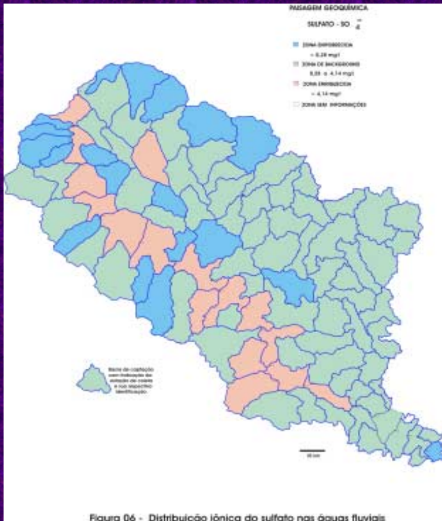
Figura 06 - Distribuição iônica do sulfato nas águas fluviais
