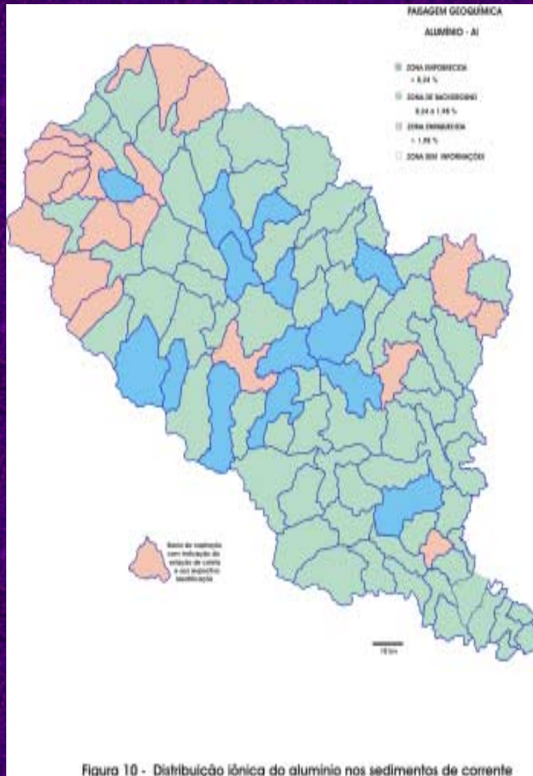
Figura 10 - Distribuição iônica do alumínio nos sedimentos de corrente
