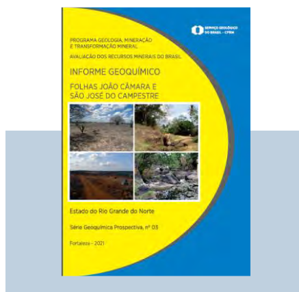
Capa do Informe Geoquímico nº 3 – Folhas João Câmara e São José do Campestre (RN).
