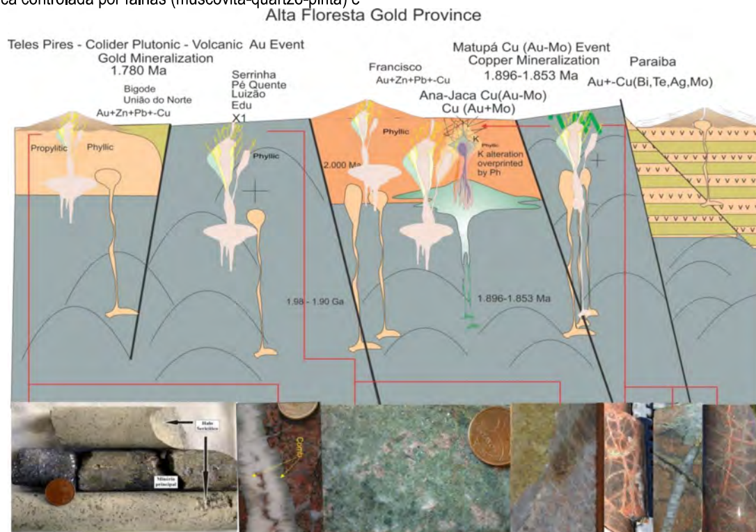
Figura 5. Imagem mostrando os eventos magmáticos e diferentes estilos de Au e Cu-Mo na PAAF. Dados geocronológicos e imagens da apresentação do Prof. Rafael Assis em 2021.
